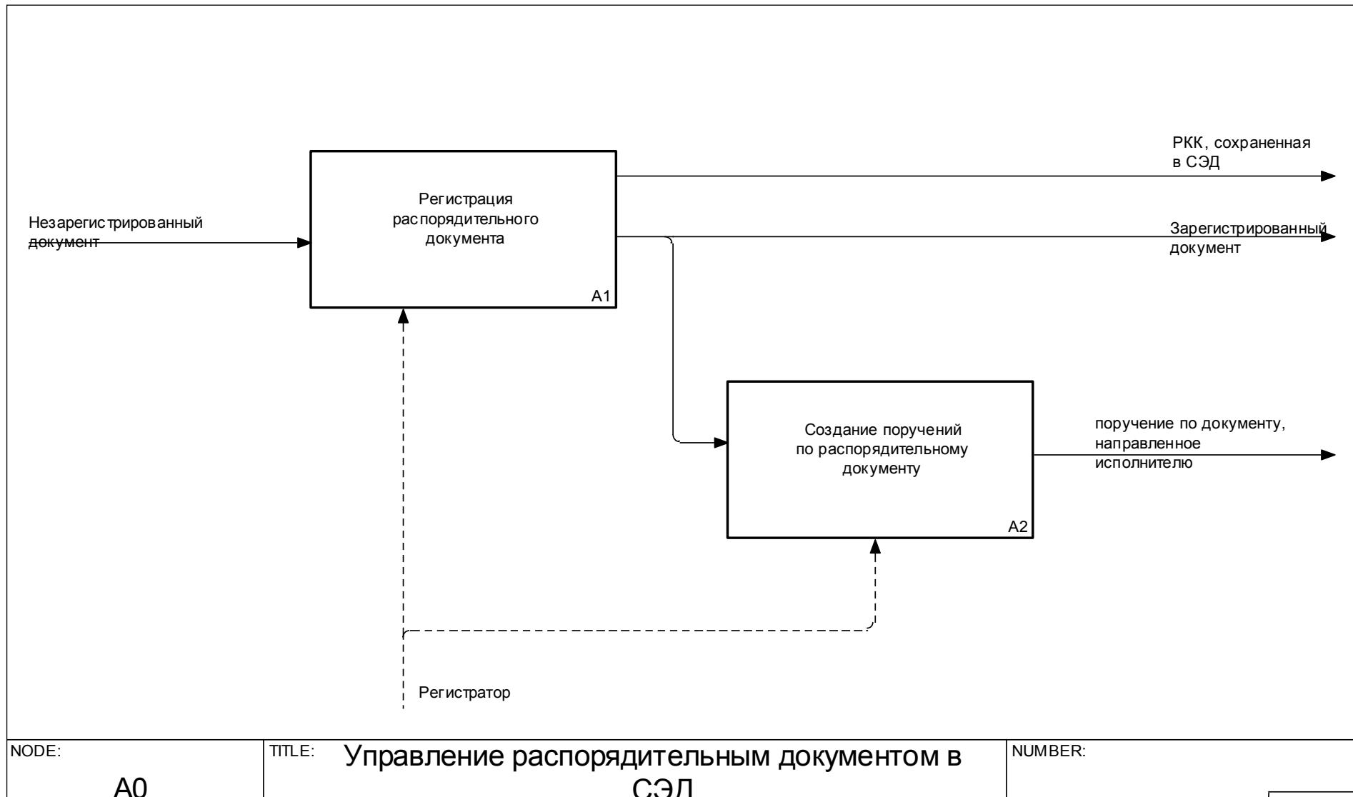
Рис.1 Управление распоряжительными документами в ESCOM.BPM
